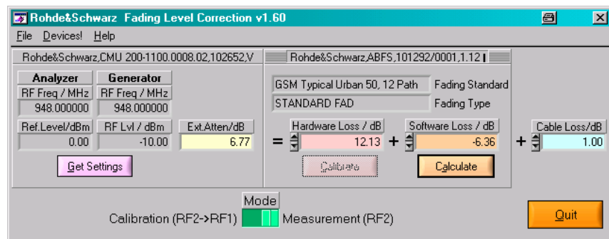
Fig. 21 GSMFadLevCor Setup
