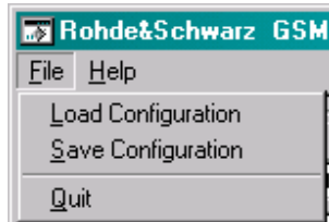
Fig. 13 Menu Items
